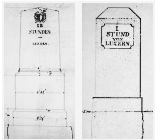
Abb.1 Entwurf für die Stundensteine an der Strasse von Luzern nach Basel und das Modell des Stundensteins von Bargezi (Stundenstein mit Walmdach). Aus Froelicher 2007, 2002, 29.
