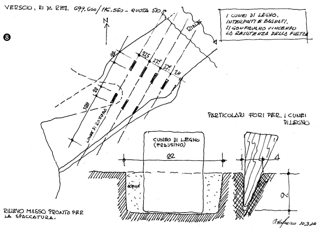
Zeichnung von O.Hofmann zum Block mit Keiltaschen
